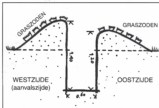
Doorsnede loopgraaf (in klei, zonder piketpalen)
