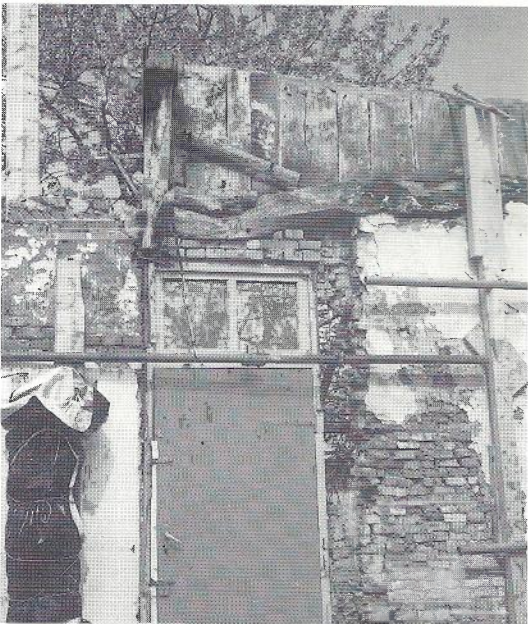
Detail voorgevel aan de binnenzijde boven de voordeur. Een gedeelte van de gebintpoot staat nog boven het kozijn van de vrij nieuwe voordeur in een kozijn uit de vroeg 20e eeuw. Hierboven de afgezaagde dekplaat, waarop de daksporen hebben gerust. Op de gebintligger staande delen hout van ong. 75cm welke aan de buitenzijde aangesmeerd zijn.
